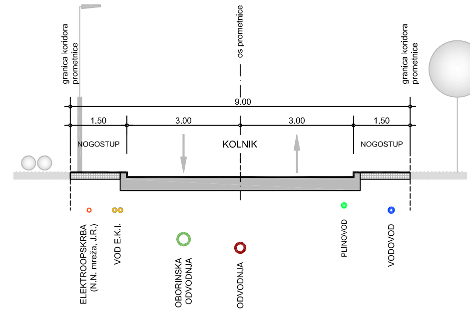
KARAKTERISTIČAN PROFIL PROMETNICE A-A (9.00 m)
